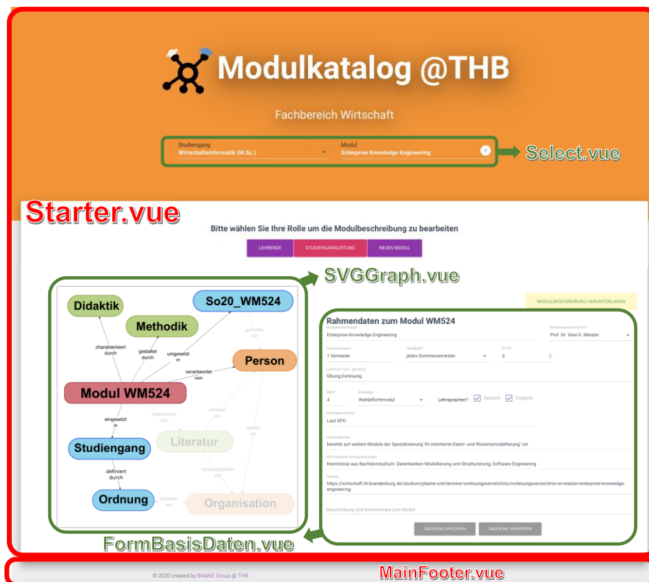
Abb. 4: User Interface mit Hervorhebungen zur Kennzeichnung der Vue-Komponenten
