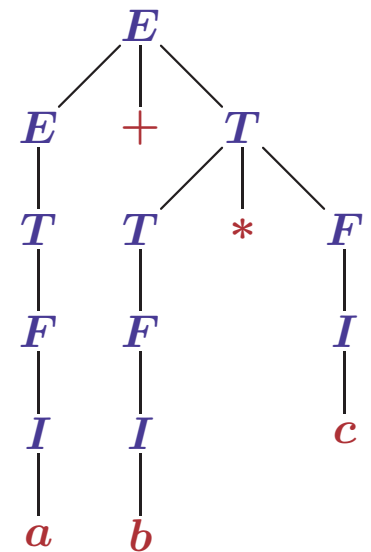
Einziger Ableitungsbaum für a + b * c
